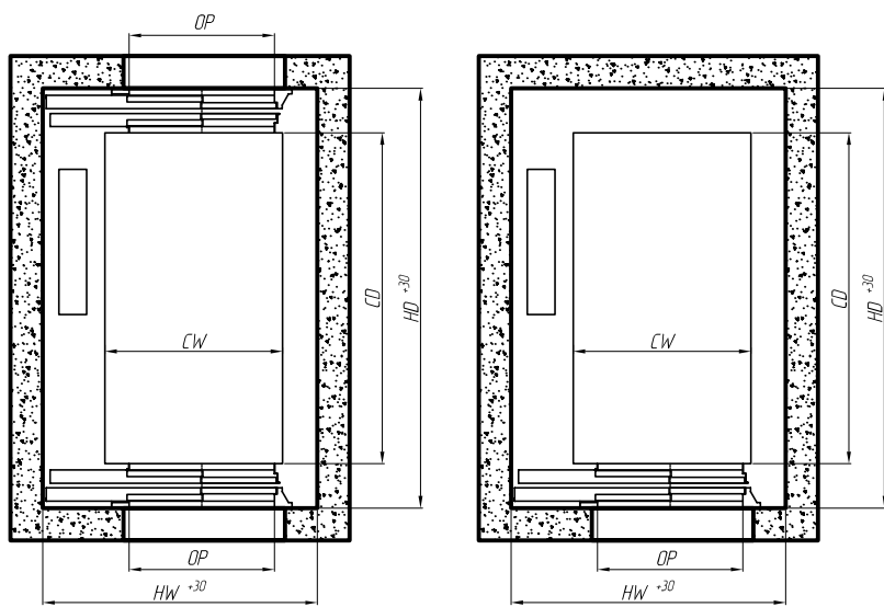
Wewnętrzne wymiary szymbów w przekroju
